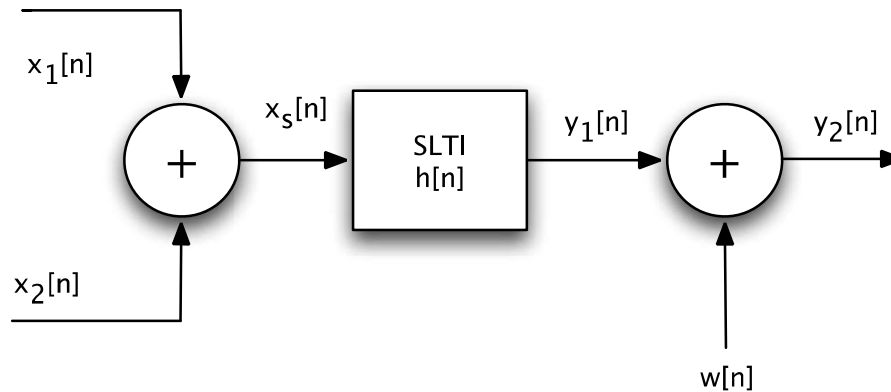
Figura 4. Esquema discreto de sistema de comunicación.
